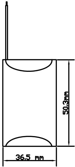
3.7V 1200mAh(1S1P)
